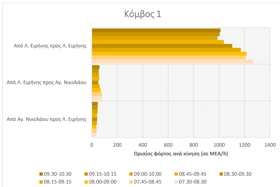
Διάγραμμα 12: Κυκλοφοριακός φόρτος ανά κίνηση στον κόμβο 1
