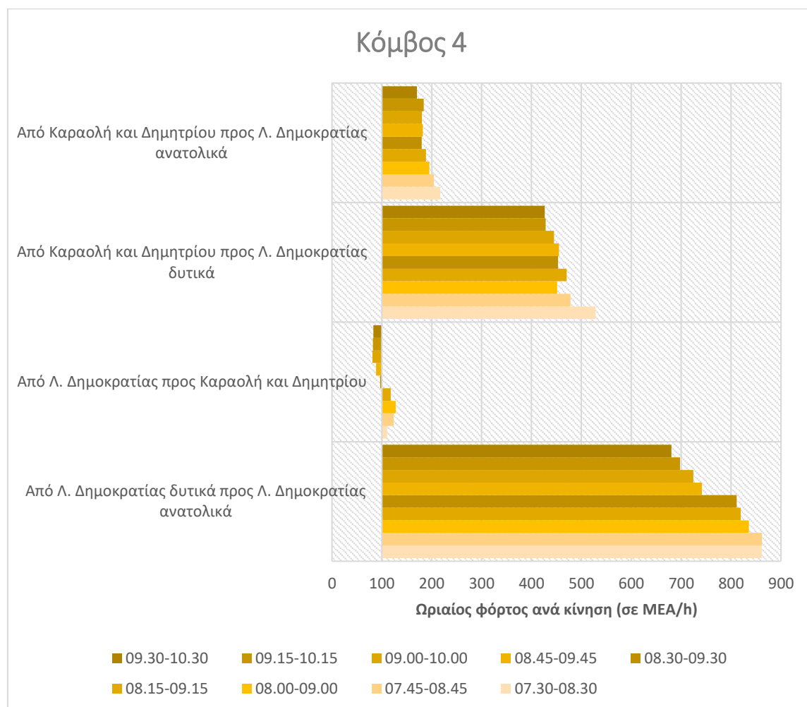
Διάγραμμα 21: Κυκλοφοριακός φόρτος ανά κίνηση στον κόμβο 4
