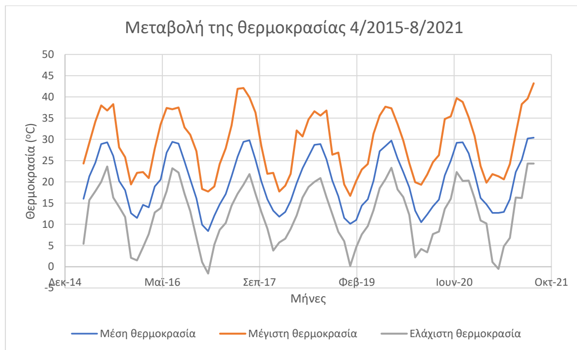
Διάγραμμα 7: Μεταβολή θερμοκρασίας Περάματος 2015-2021
