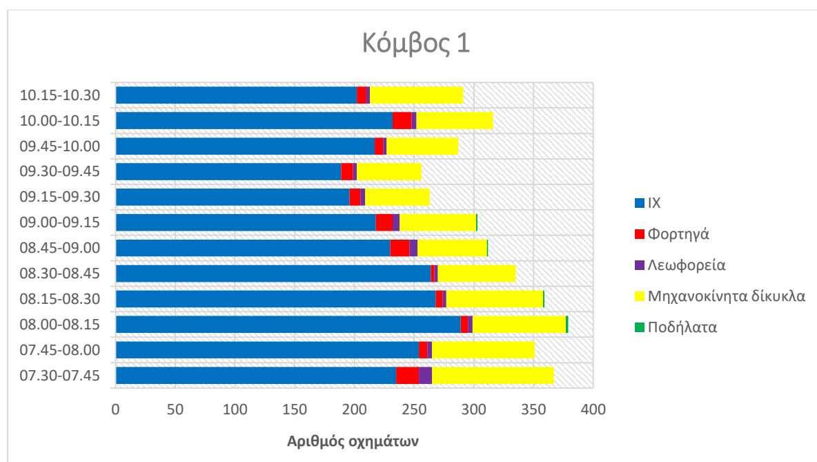
Διάγραμμα 11: Σύνθεση κυκλοφορίας ανά χρονική μεταβολή κόμβου 1
