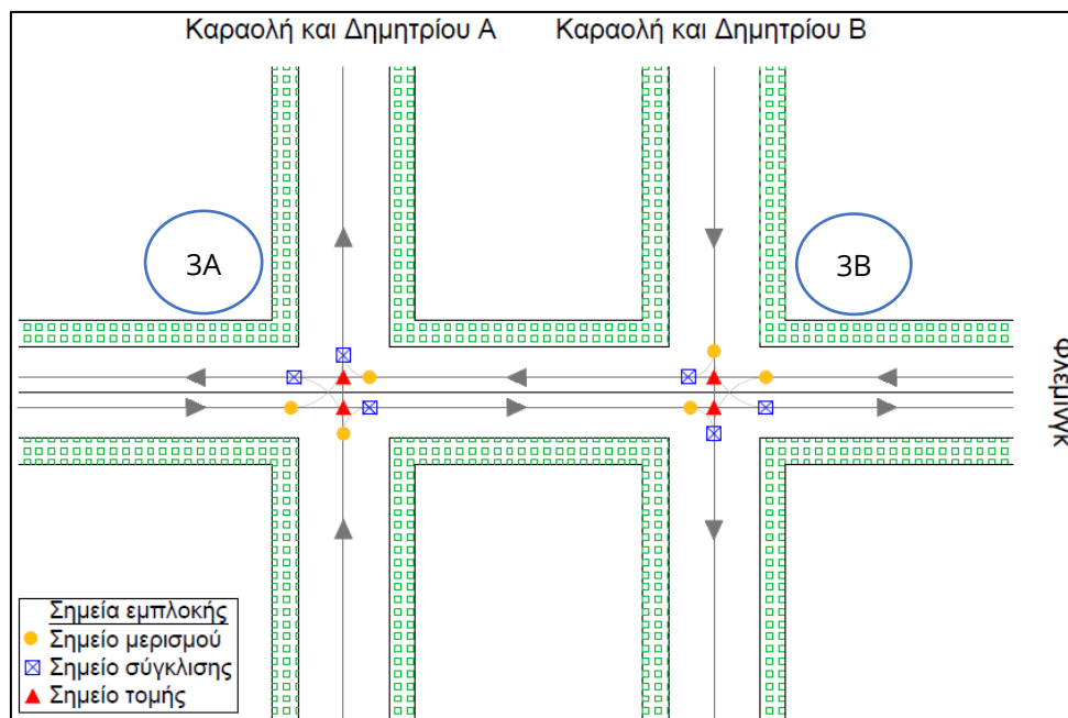
Εικόνα 53: Παρουσίαση σημείων εμπλοκής στον κόμβο 3 (Πηγή: επεξεργασία αναδόχου)
