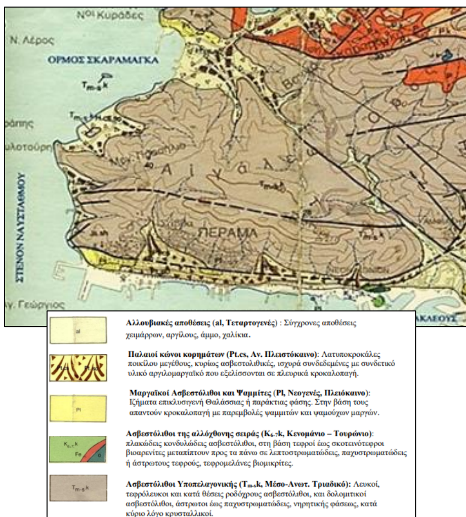
Εικόνα 45: Απόσπασμα γεωλογικού χάρτη Ι.Γ.Μ.Ε, φύλλο Αθήνα-Πειραιάς
